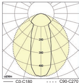
MASTIF-T70, 2x36W, IP54
