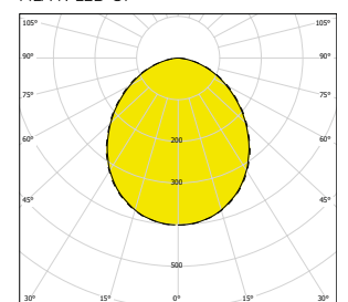
FILA-N-LED-OP
